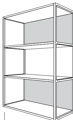
Moduł 30H z plecami tapicerowanymi B3 231
