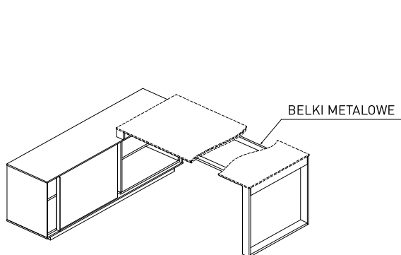
PRZYKŁADOWE WYKORZYSTANIE KOMODY PODBIURKOWEJ
