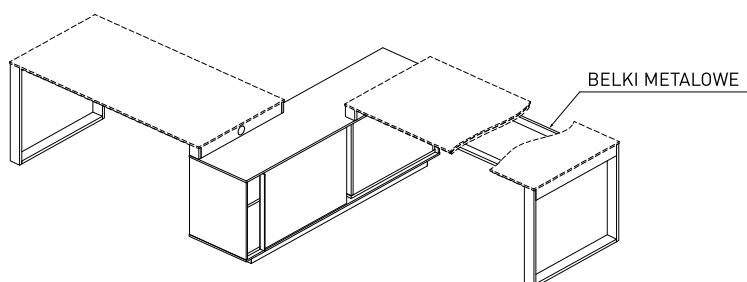
PRZYKŁADOWE WYKORZYSTANIE KOMODY PODBIURKOWEJ DLA DWÓCH BIUREK
